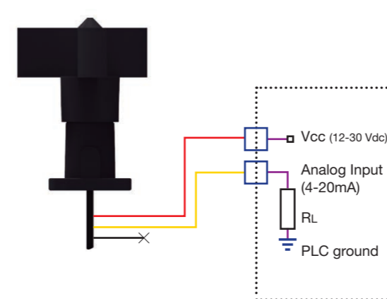
ANEMO4403 V3 4-20 mA OUTPUT
